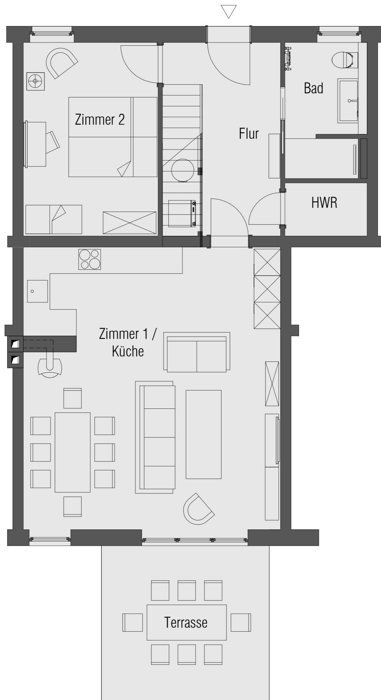
Grundriss Erdgeschoss
